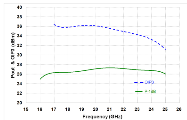
Pout +IP3
