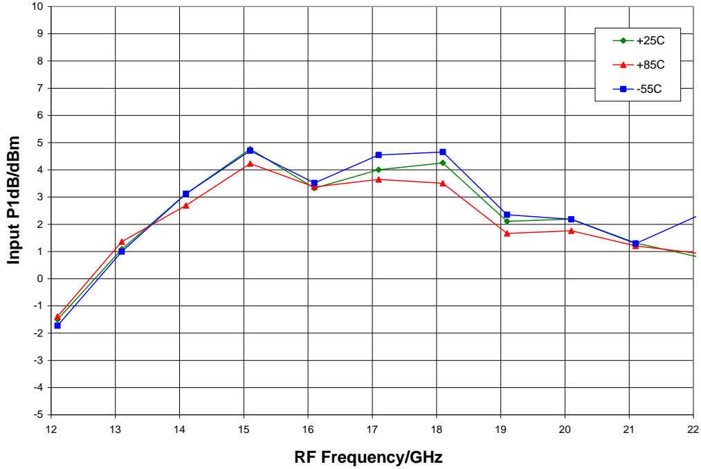
Input P1dB vs. Temperature, LO = +2 dBm
