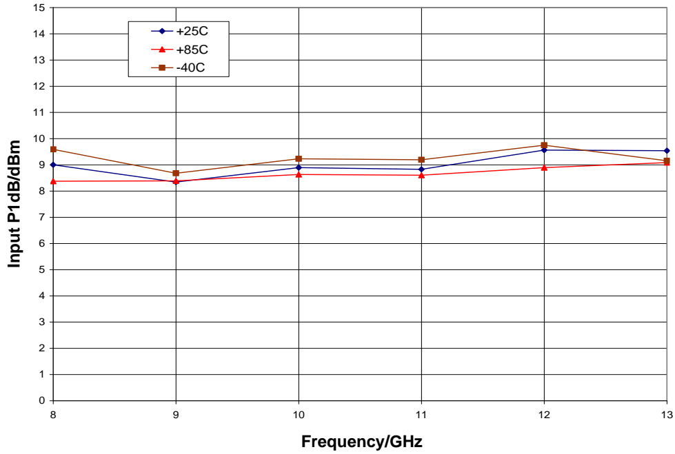
Input P1dB vs. Temperature, LO = +15 dBm, IF = 100 MHz USB
